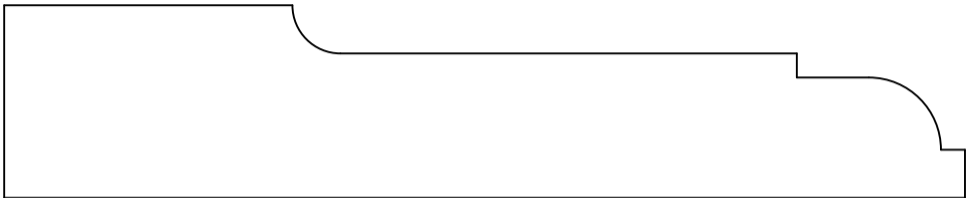
HWP7398 Molding 1.000" x 5.000"
