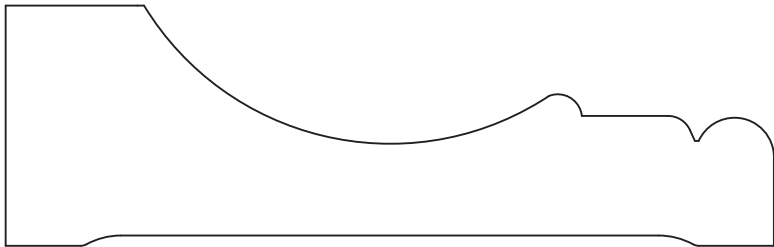
HWP4191 Apron 1.250" x 4.000"
