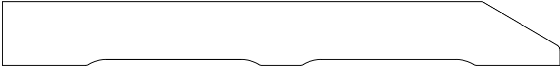
hwp3118_Base 0.687" x 6.000"
