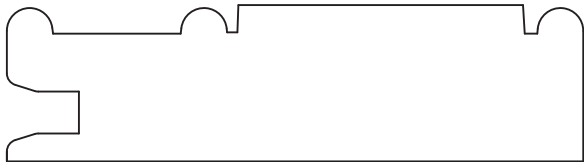
9763 Frame 0.812" x 3.000"
